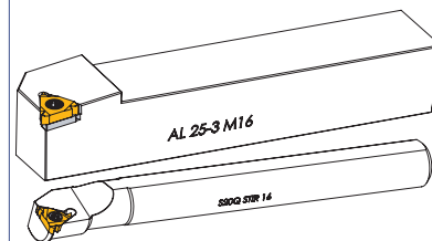
Державки расточные 61-71
