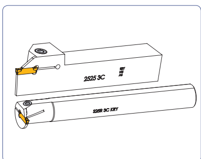
Державки канавочные 100-105 /107-109
